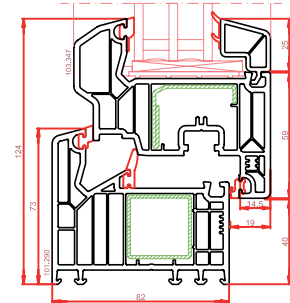
SECCIÓN VERTICAL
